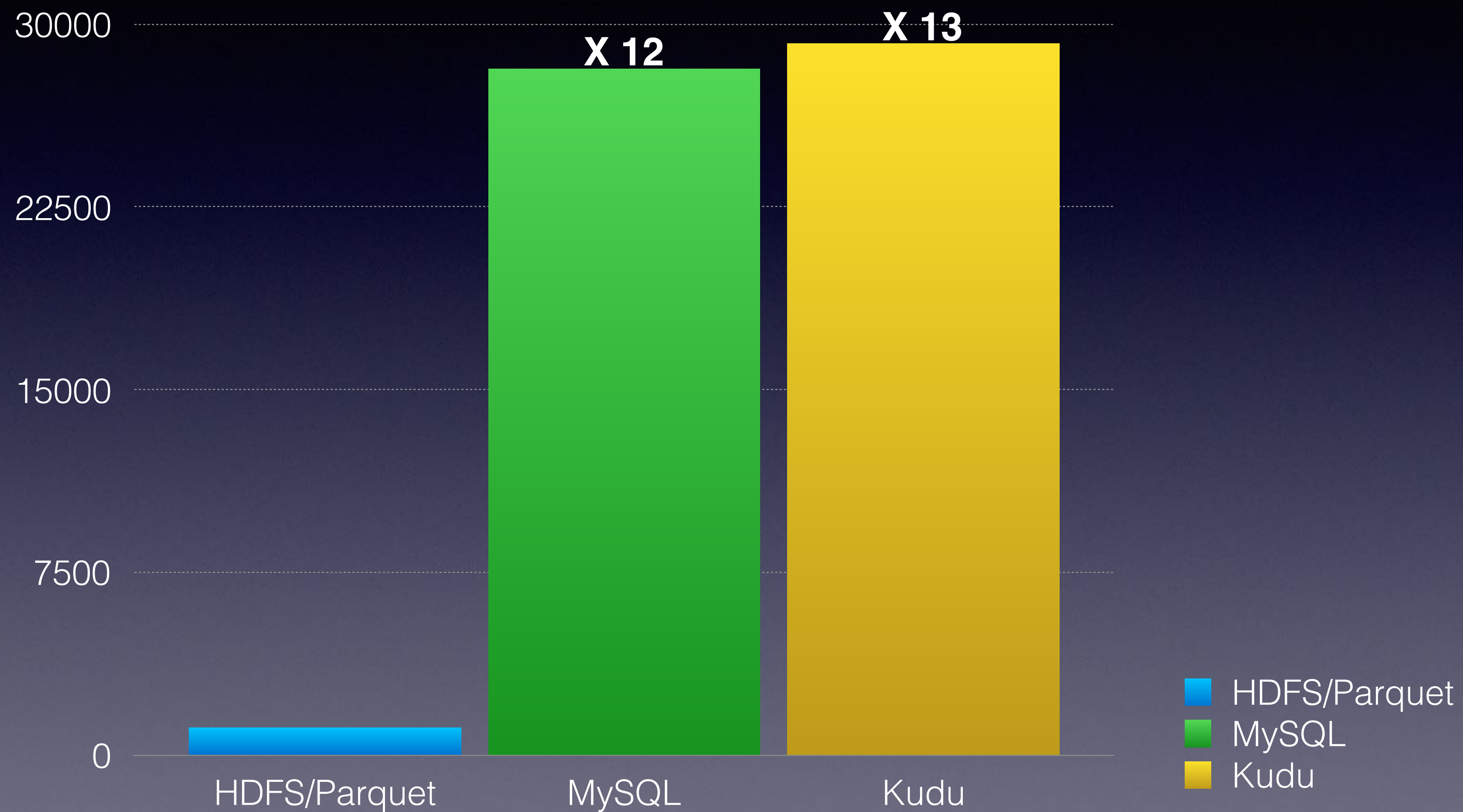
Kudu 性能对比 – 随机写入 (62GB)
